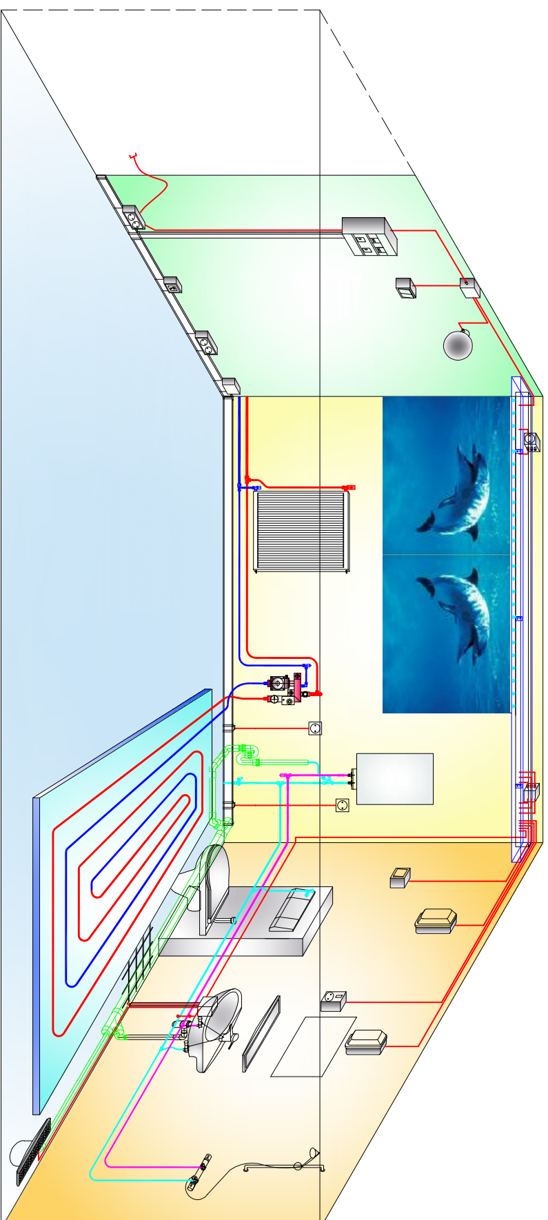
Indeling dagverblijf voor de trainers van het dolfinarium
